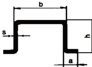
HUT-Profil "HNP"
